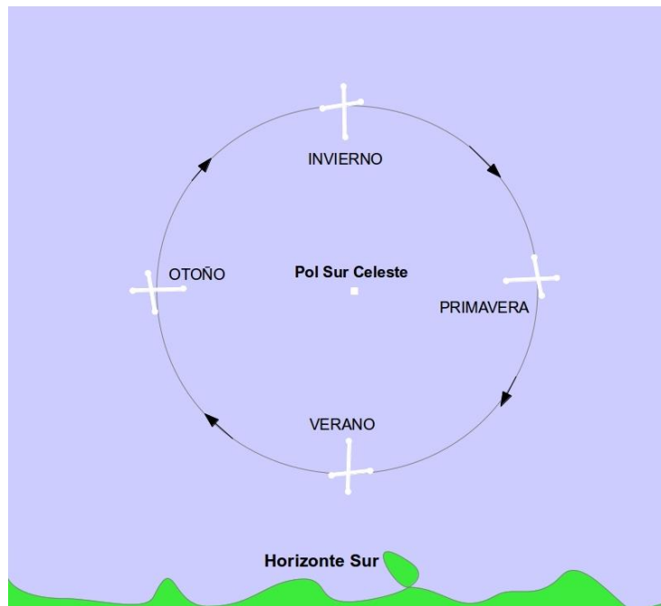
Fig. 11: Posiciones relativas de la Cruz del Sur en torno al polo sur a lo largo del año (a la misma hora).
