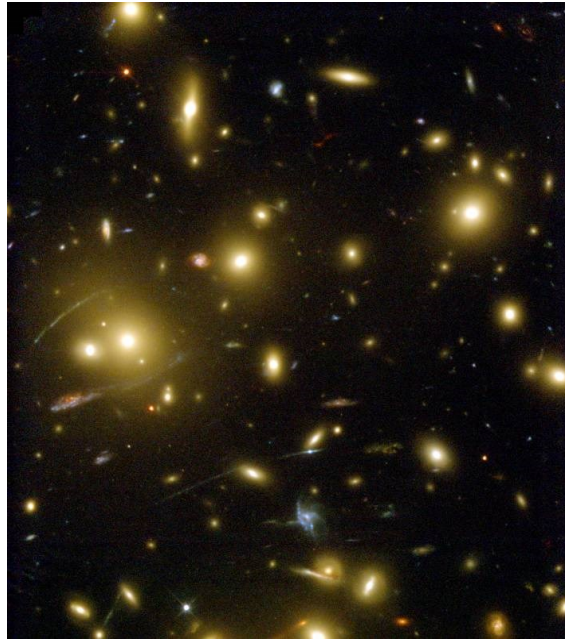
Fig. 3: Cúmulo de galaxias Abell 2218 Se pueden distinguir arcos derivados del efecto de lentes gravitacionales. (Foto: NASA, ESA, Richard Ellis (Caltech) and Jean-Paul Kneib (Observatoire Midi-Pyrenees, France)).
